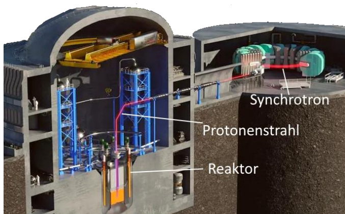
Abbildung 5: Transmuter - Reaktorprinzip
