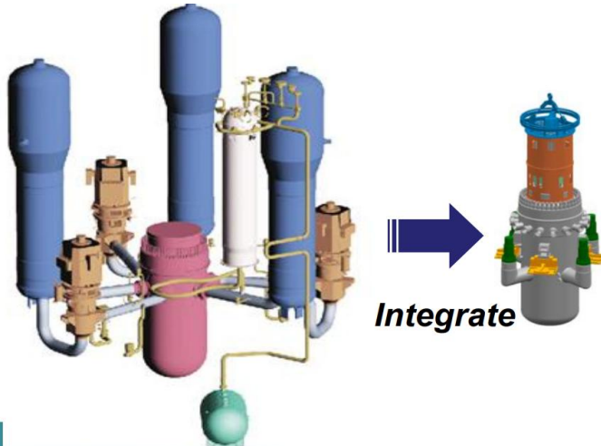
Abbildung 7; Prinzip des Chinesischen ACP100
