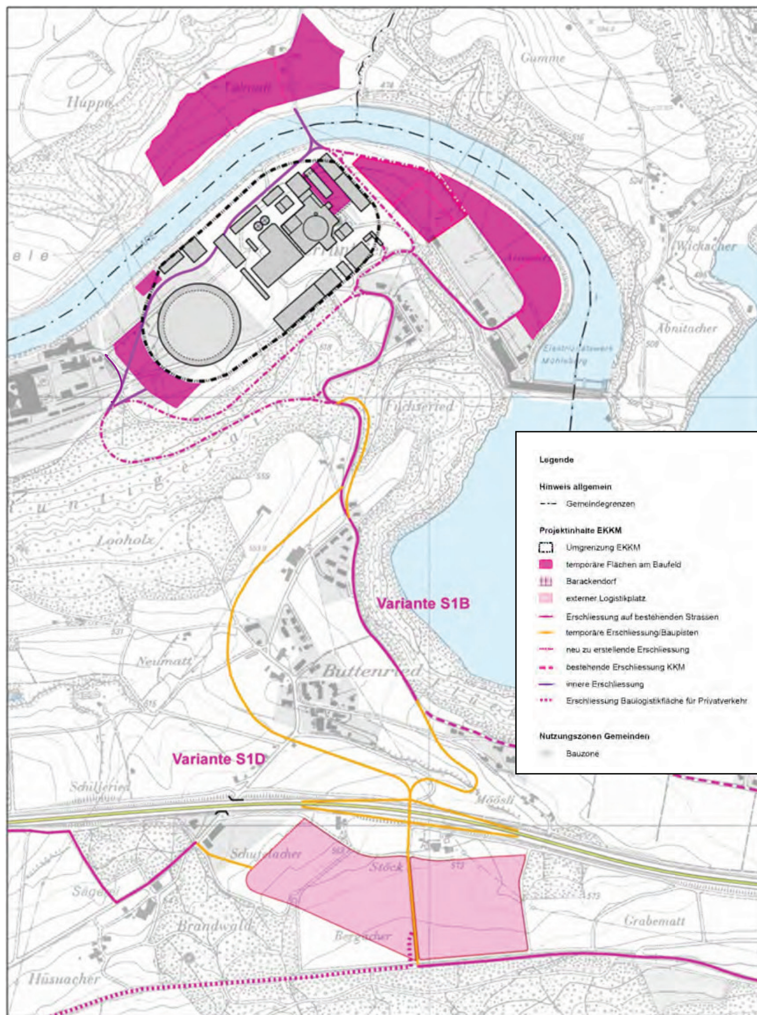
Abb. 3.4-1: Erschliessungsvarianten Strassen
